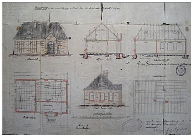
Tegning til den nye skolebygning.
