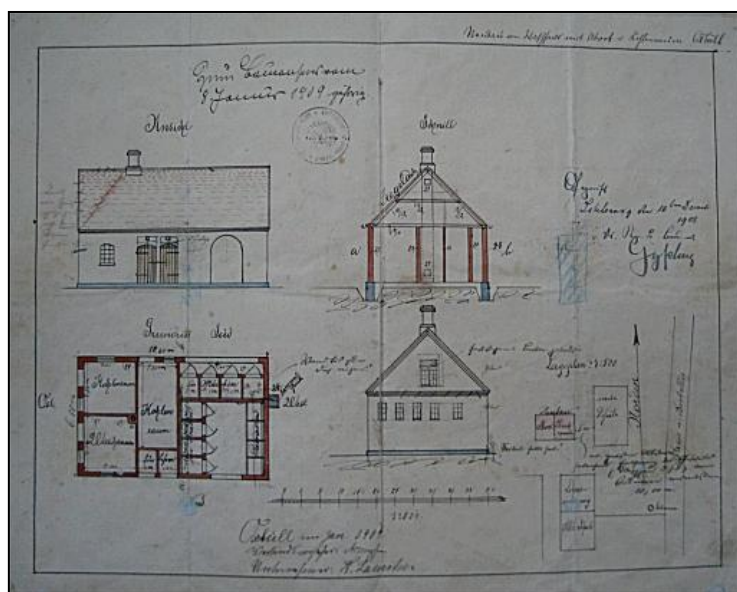
Tegning til det nye vaskehus med toilet og kul rum.
