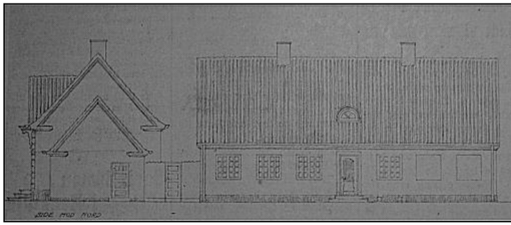
Tegning af den nye skole set fra nordsiden.
